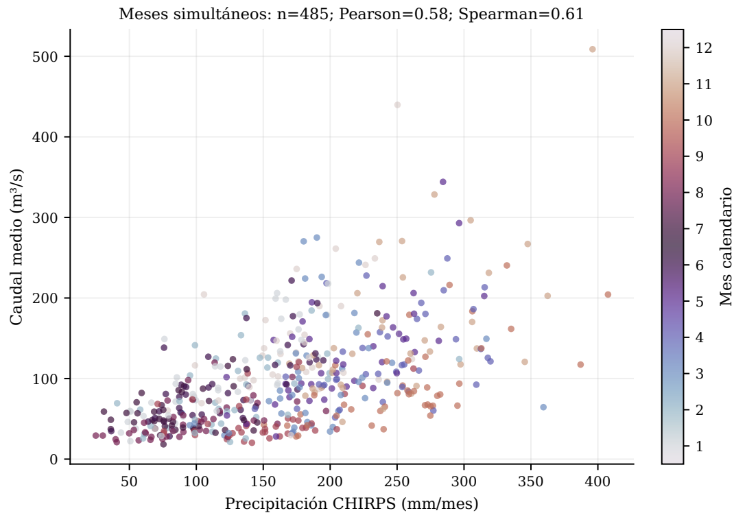
Figura 23: Relación descriptiva entre precipitación CHIRPS y caudal, sin rezago.
