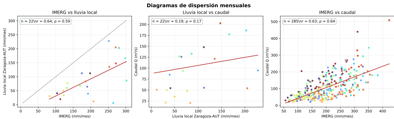
Figura 22: Diagramas de dispersión requeridos. La línea discontinua en IMERG–lluvia local es 1:1.
